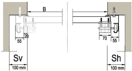
LHR FM architrave ribassato doppia guida, molle frontali
