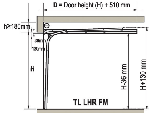
LHR FM architrave ribassato doppia guida, molle frontali
