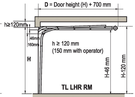
LHR RM architrave ribassato doppia guida, molle posteriori
