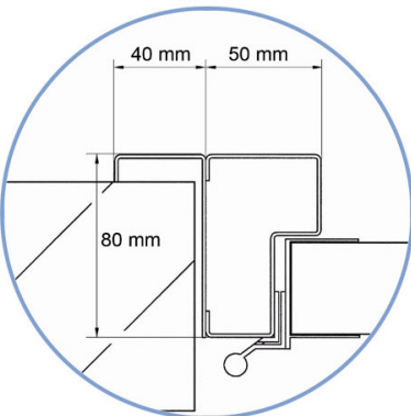
Layout telaio
